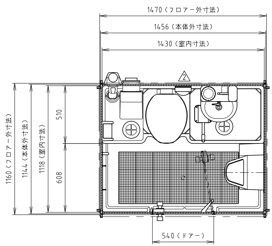
平面図 (内装)
