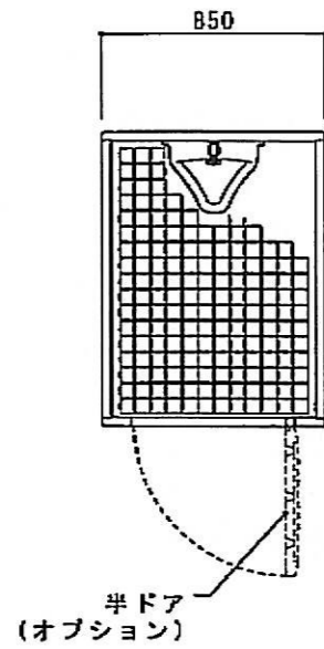
平面図 S=1/30
