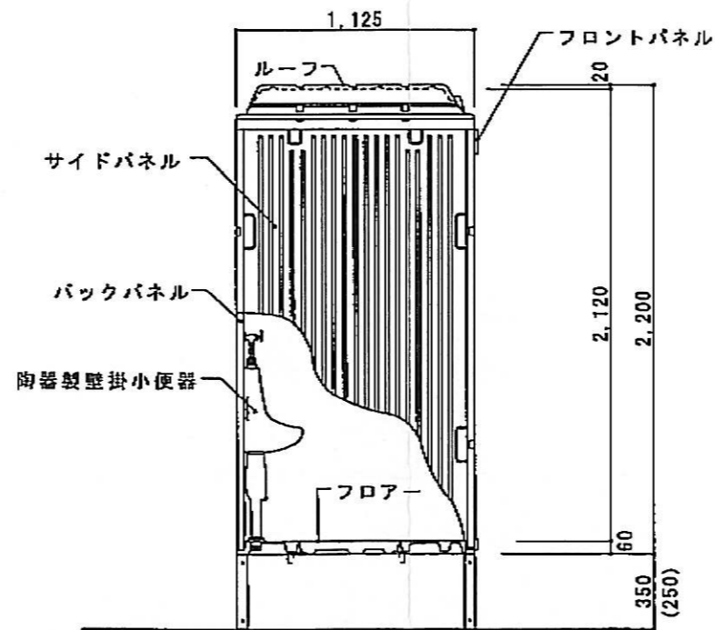
断面図 S=1/30
