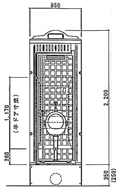
A 立面図 S=1/30
