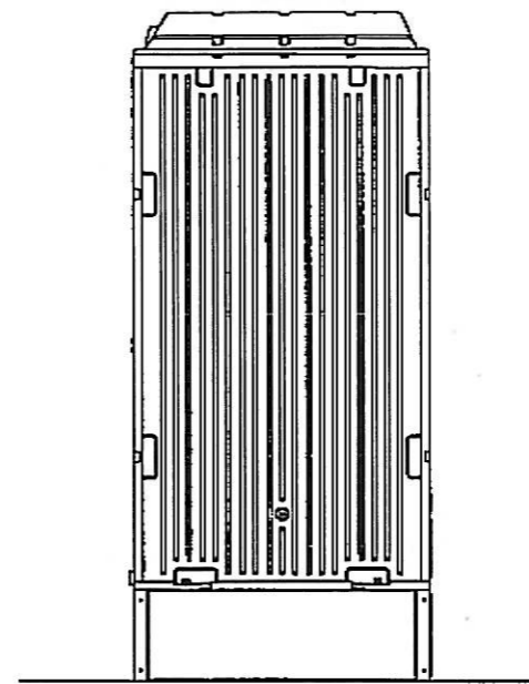
D 立面図 S=1/30
