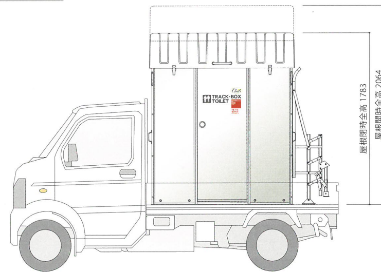
軽トラック積載時全高2500未満(道路交通法)
