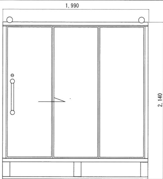
正面図
