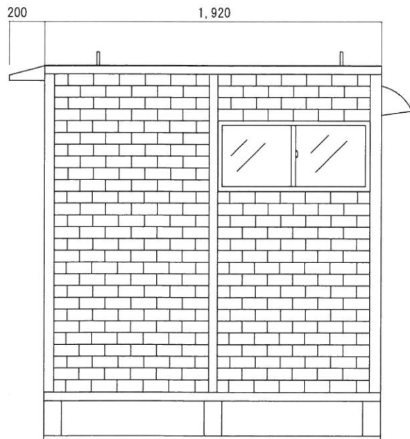
右側面図
